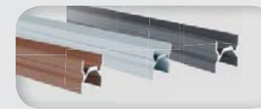
Należy montować jedną listwę pośrednią co trzy deski. Wymiary w mm: 23,3x24x1730 (dla wykończenia gładkiego). 23,3x24x1736 (do wykończenia piaskowanego).
