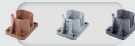
Wymiary w mm: 27x9,5x1815 (z wykończeniem gładkim i z wykończeniem piaskowanym).
